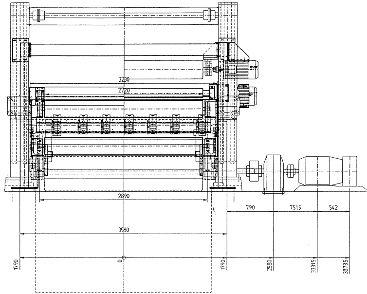
LEIKKAUS A-A
