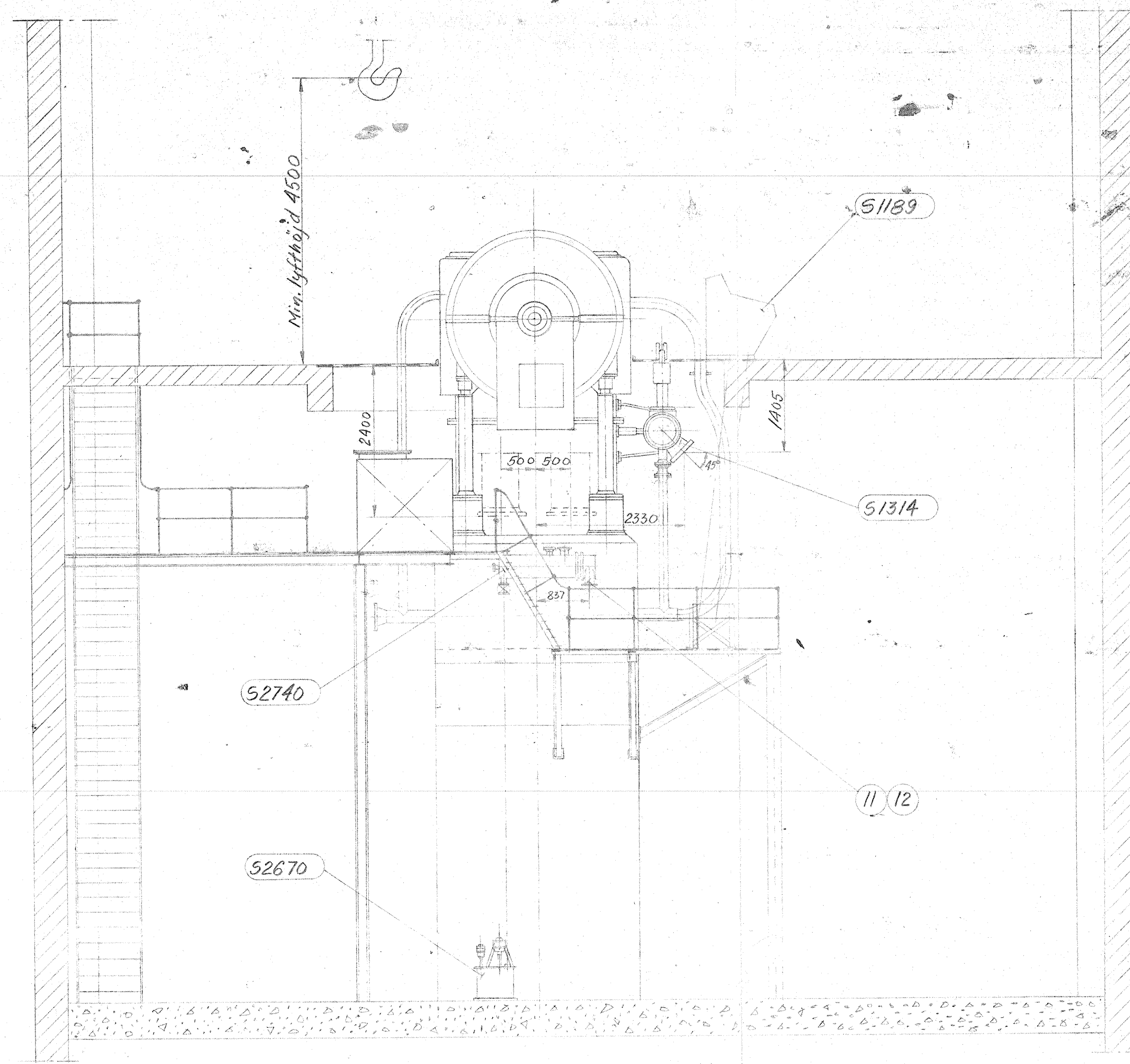
Sekt. B-B
